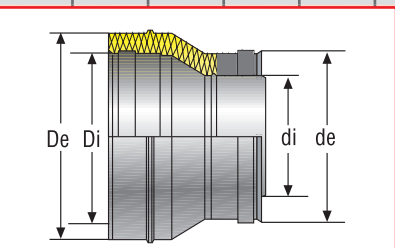
ÉLÉMENT DP RÉDUIT MALE DP VERSMALD BUSTEKKERVORMIG ELEMENT DW
