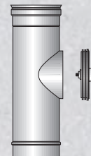
RACCORD ENCOMBREMENT VISITE RÉDUIT VERKLEIND INSPECTIE VERBINDINGSTUK
