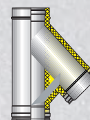
RACCORD EN T 135° DP
