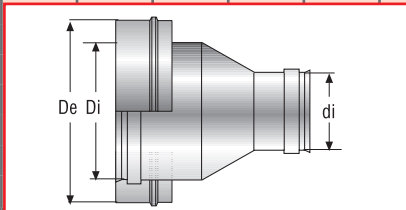
ÉLÉMENT FERMETURE DP RÉDUIT SIMPLE FEMELLE VERSMALD ENKELVOUDIG BUSVORMIG SLUITELEMENT DW
