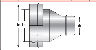
ELEMENT FERMETURE DP REDUIT SIMPLE MALE VERSMALD ENKELVOUDIG STEKKERVORMIG SLUITELEMENT DW
